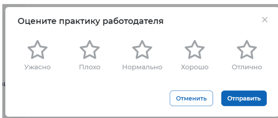
Рисунок 33 – Выбор оценки
