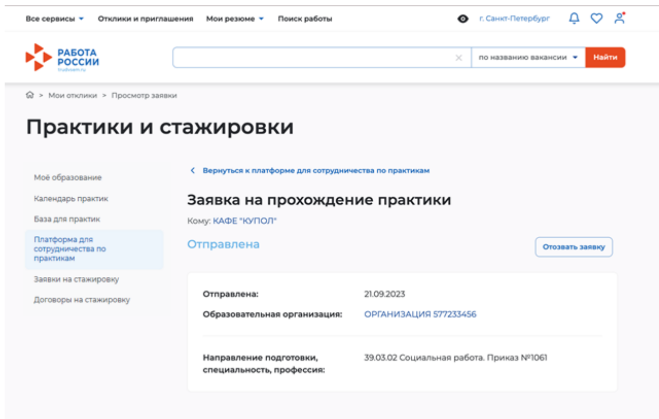
Рисунок 11 – Карточка заявки
