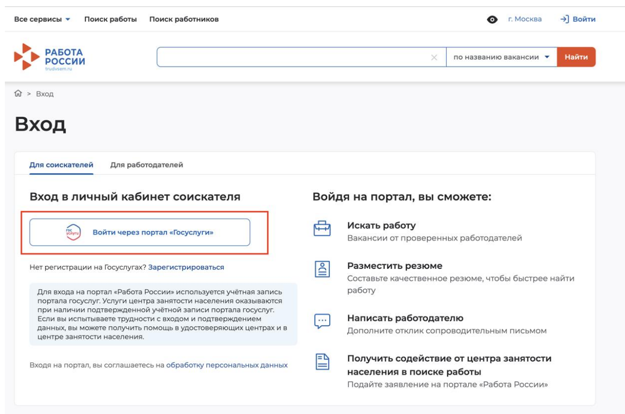
Рисунок 2 – Страница авторизации
