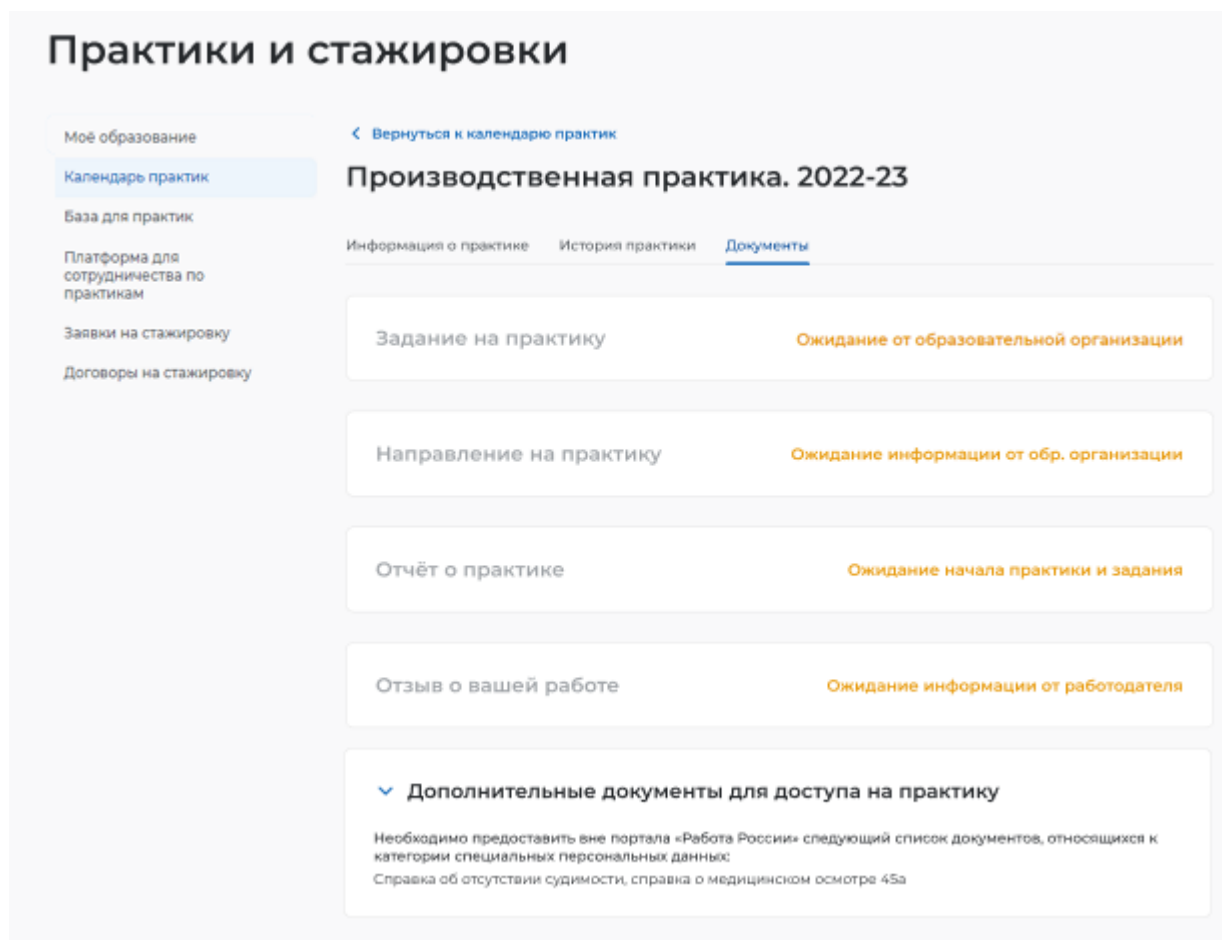
Рисунок 23 – Вкладка «Документы»
